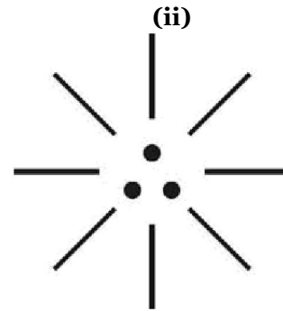
(Fundamental Neutrinos)
